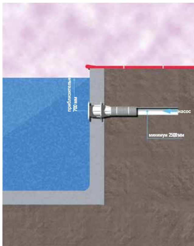
УСТАНОВКА ФОРСУНКИ
