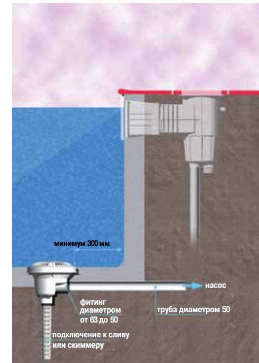
УСТАНОВКА ДОННОГО СЛИВА
