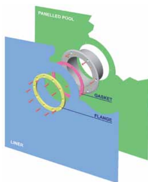
1 прокладка
