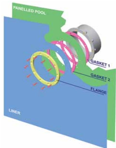
2 прокладки
