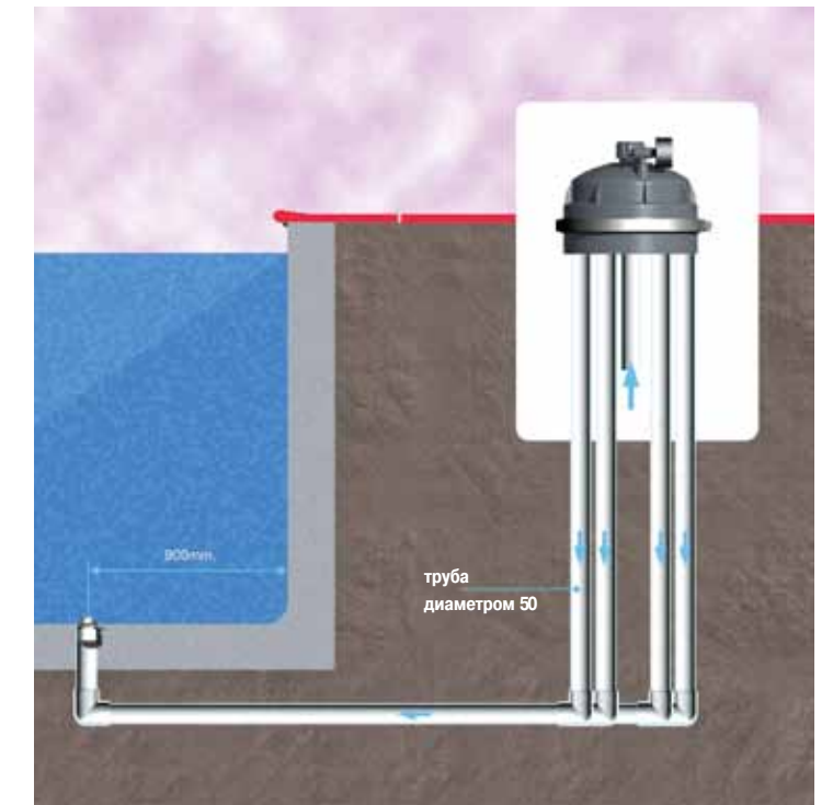
УСТАНОВКА ВЕНТИЛЯ NET'N'CLEAN
